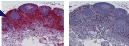
RNAscope™
